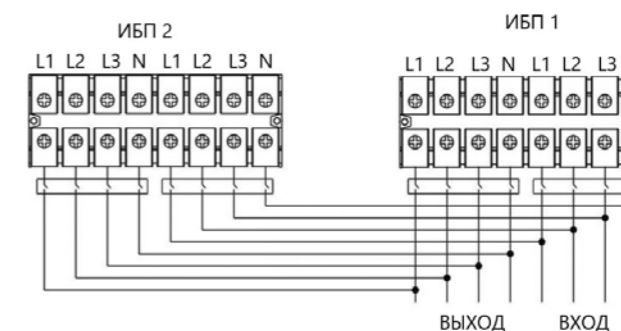
Монтажная схема параллельной системы для 15000
