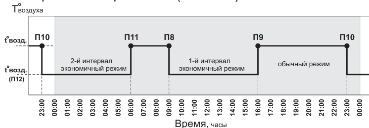
Рис.4 График температуры воздуха в помещении для Режим 1.
