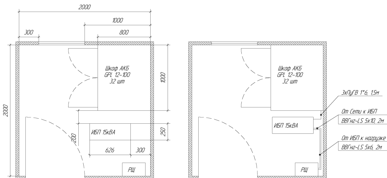
Рисунок 2 – пример проекта размещения оборудования в помещении где РЩ – распределительный щит, в котором установлены коммутирующие защитные устройства для подключения Сети к ИБП, ИБП к нагрузке
